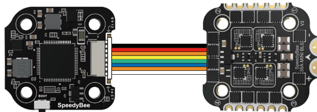
F405 Mini Flight Controller
